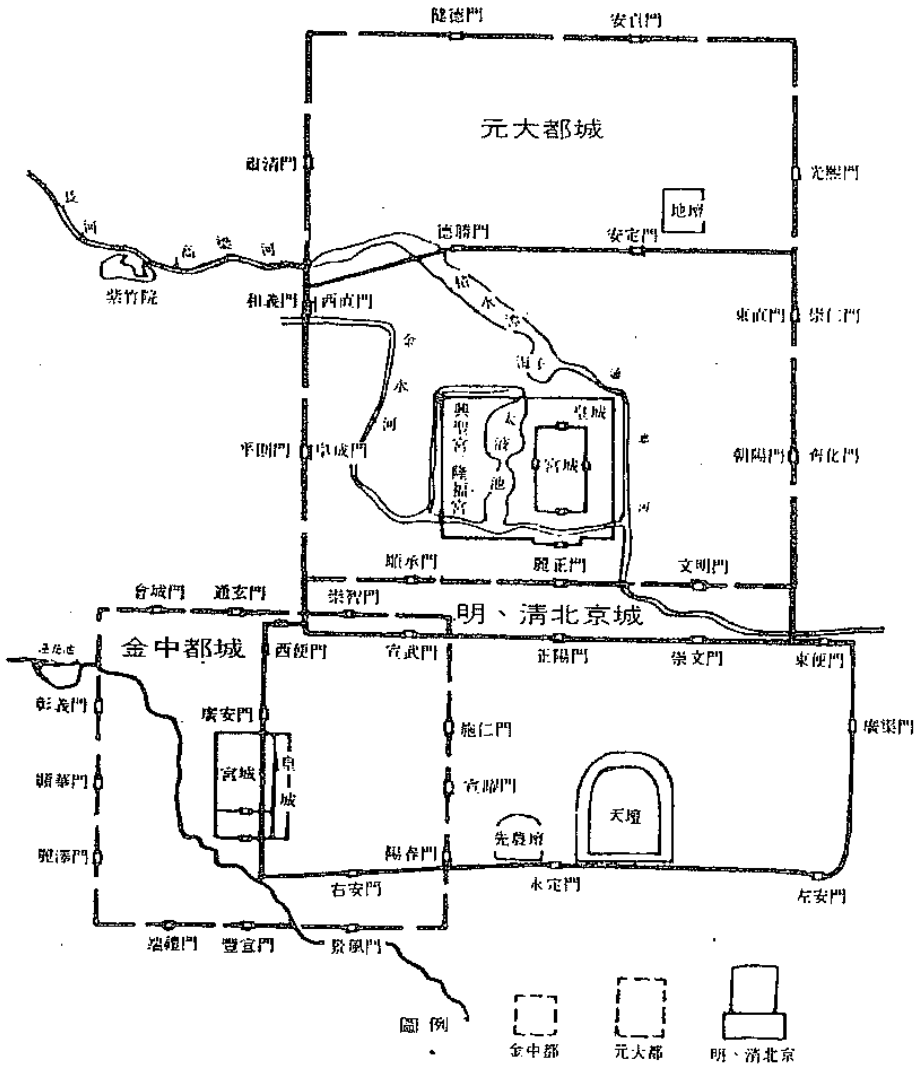
北京沿革圖
