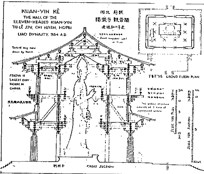
獨樂寺觀音像，遼，約西元九八四年。大慈大悲的觀音菩薩是信徒最多的一位佛教神祇。此尊觀音高十六公尺，供於純以木造的獨樂寺。橫切面由著名建築史學者梁思成繪製。
